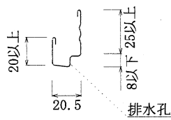
断面詳細図
