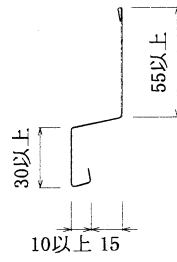
断面詳細図
