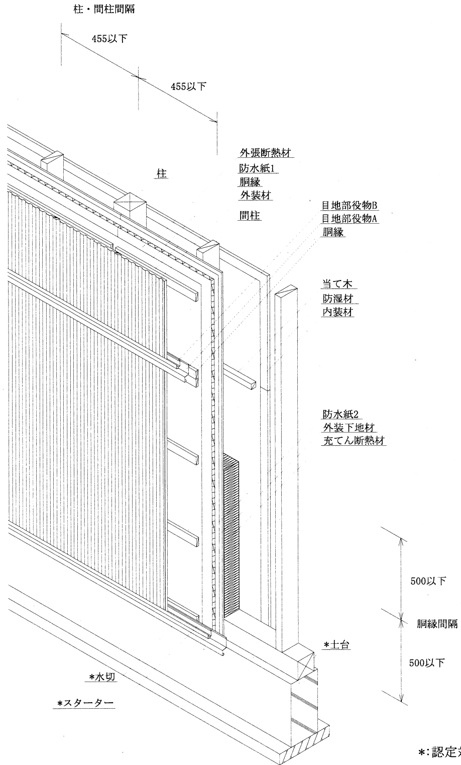
透視図 (別添-16)
